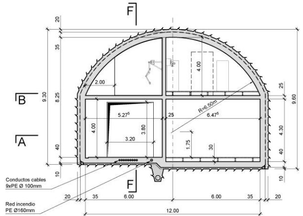
Corte D-D, 1:100
