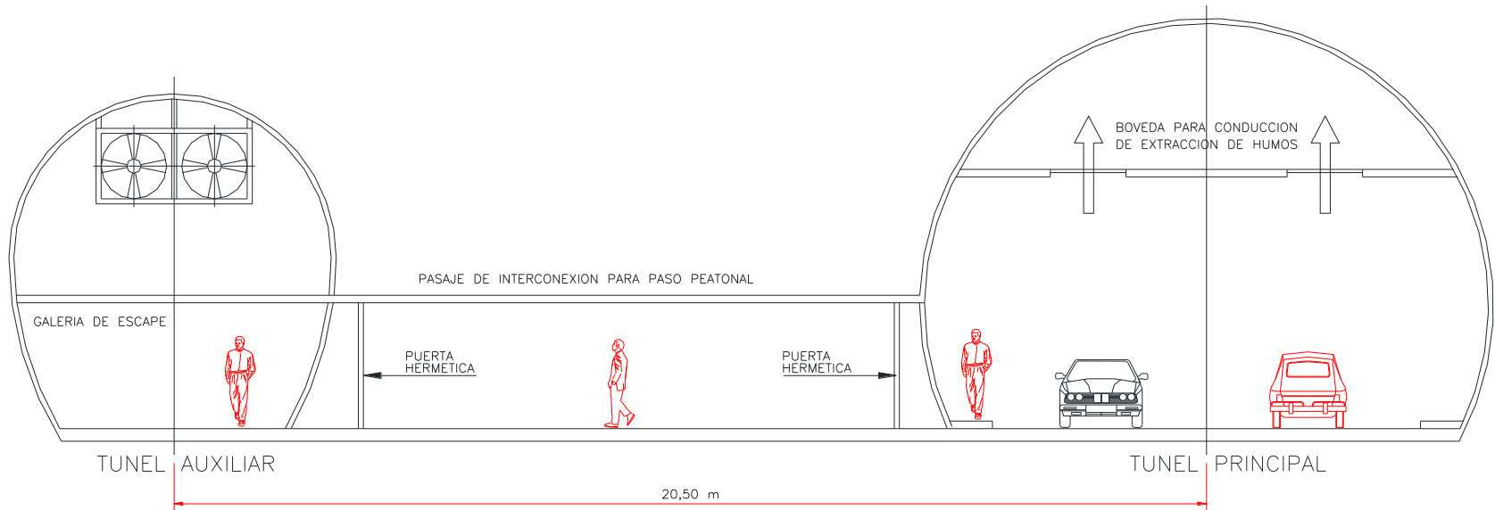
SECCION TIPICA DE LOS PASAJES DE INTERCONEXION PARA PASOS PEATONALES
