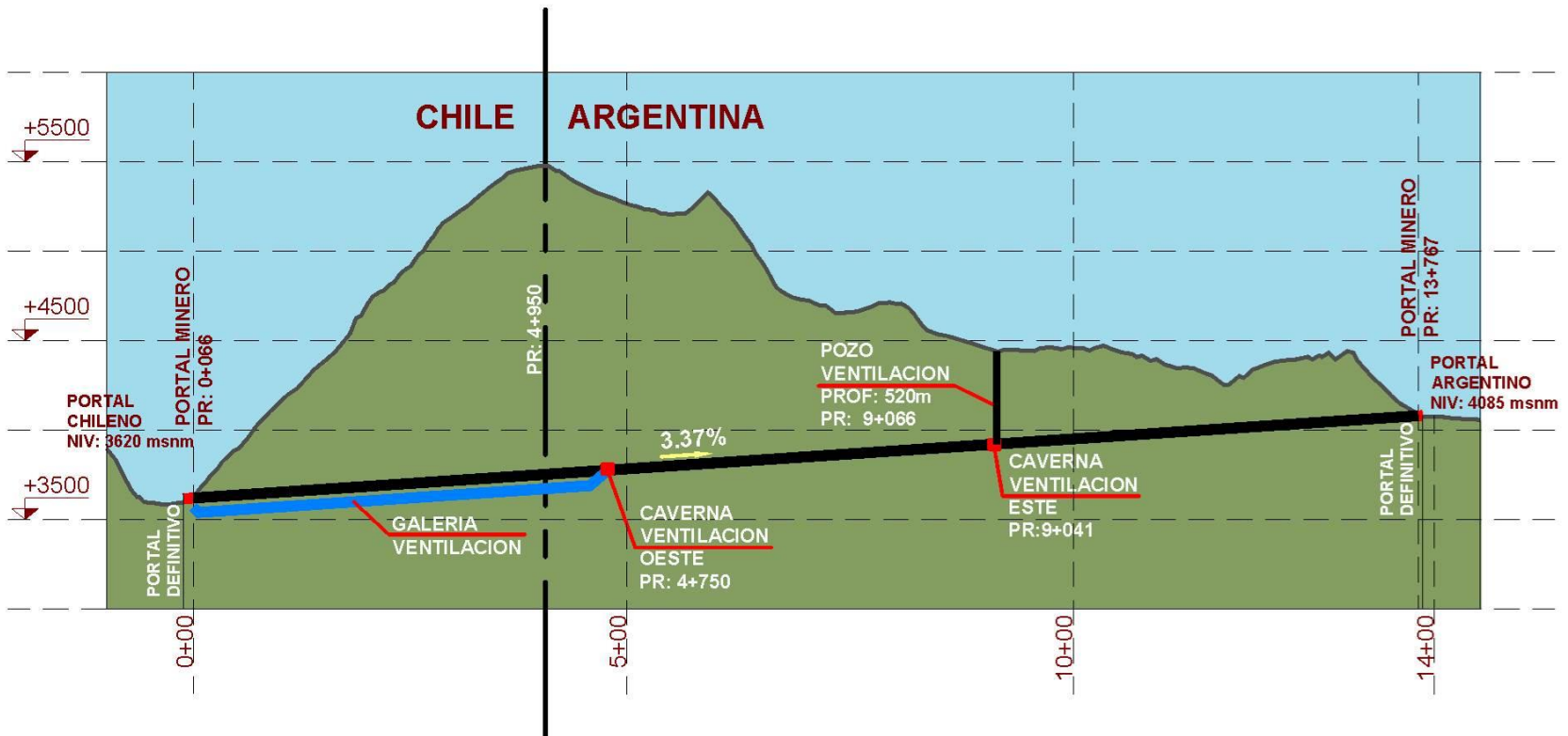
Perfil Longitudinal del Sistema
