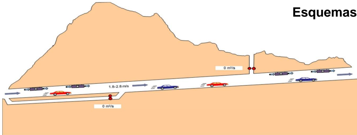
Esquema ventilación con operación normal
