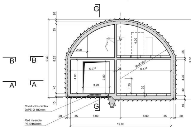
Corte G-G, 1:100
