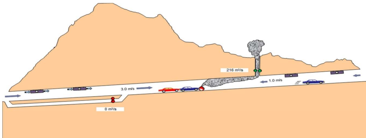
Esquema ventilación con escenario de incendio en el centro del túnel
